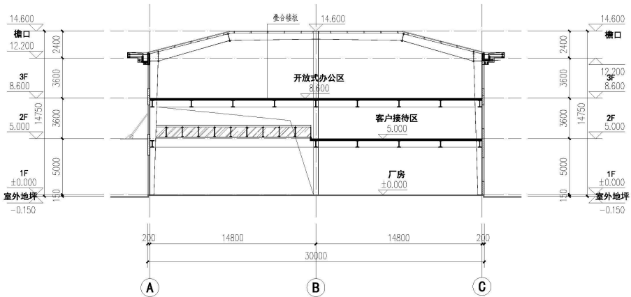
1-1 剖面图 1:200
