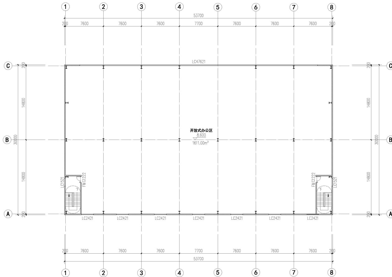
三层平面图 1:200
