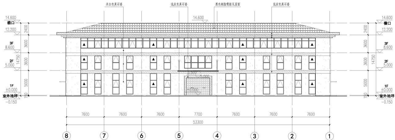
8~1 立面图 1:200
