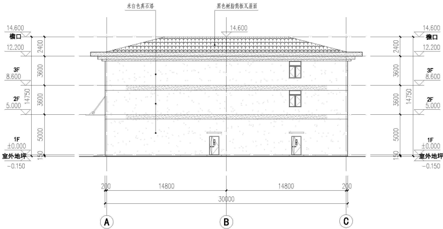
A~C 立面图 1:200
