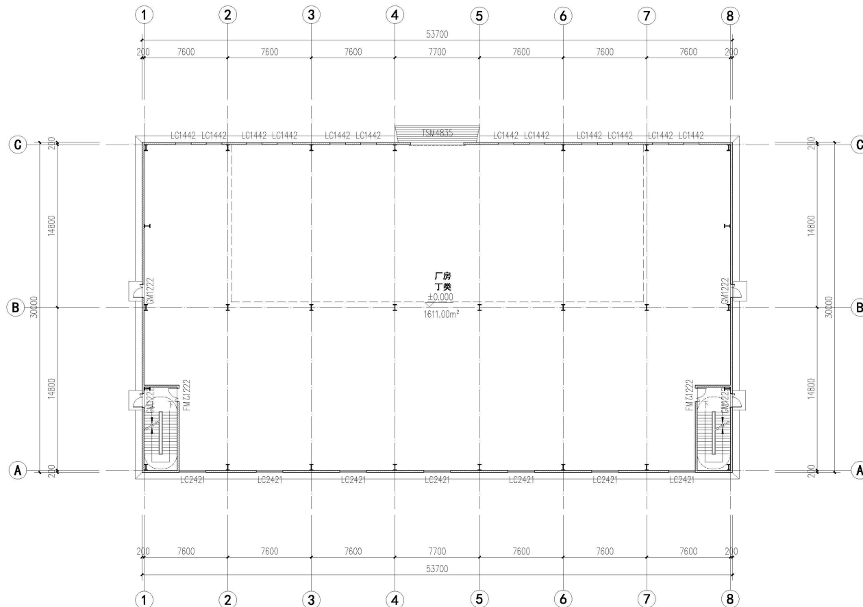
一层平面图 1:200
