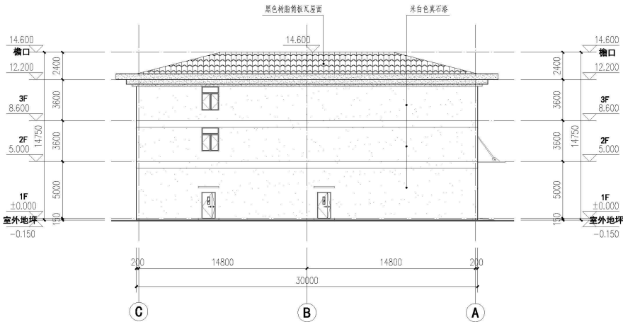
C~A 立面图 1:200
